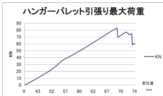
平均破壊荷重82.9kN 安全率5以上
