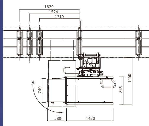
設置図
