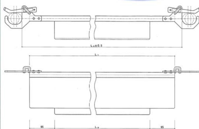
仕様 建柱足場(φ42.7mm)用
