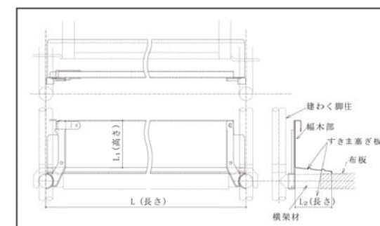
寸法図 建柱横架材取付型
